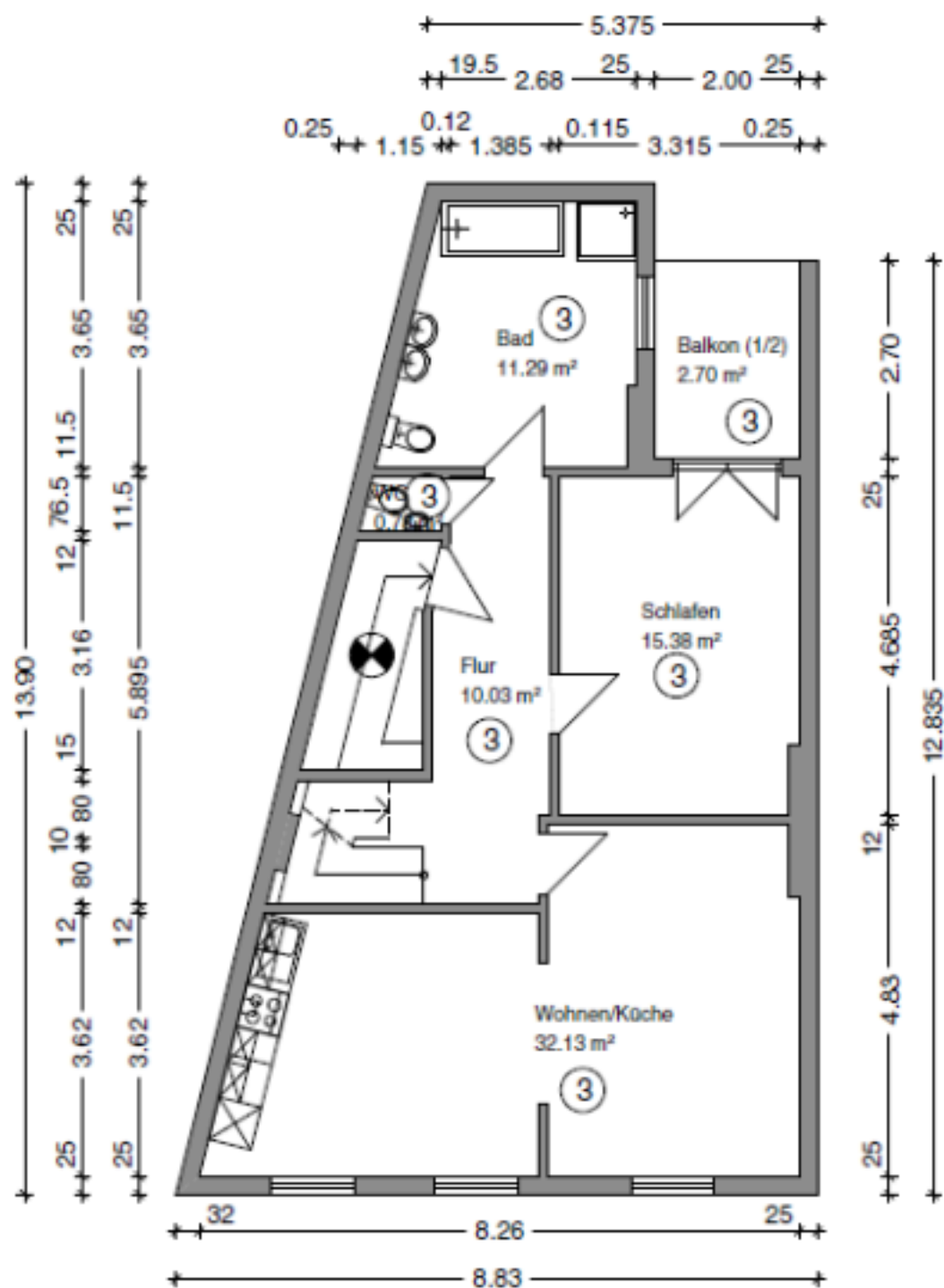
GRUNDRISS 2.OG
